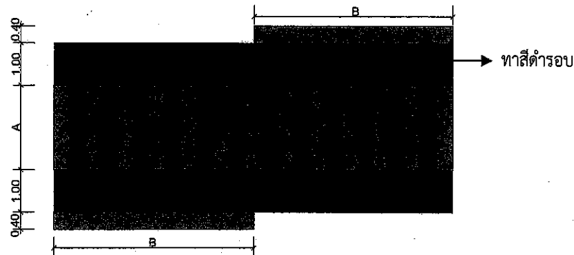
ภาพปัญหาการซ้อนทับของทางข้ามม้าลายเดิม และทางข้ามม้าลายใหม่ บนผิวแอสฟัลต์ติกคอนกรีต
